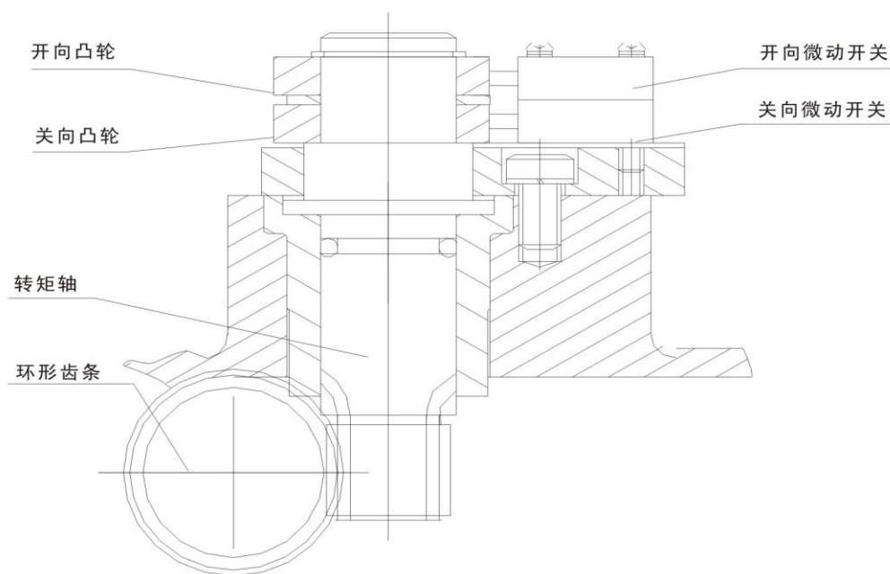
图3 转矩控制机构
