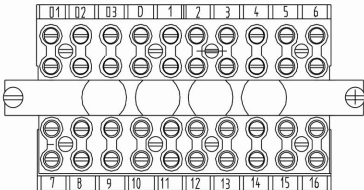
图6-1 普通型端子图
