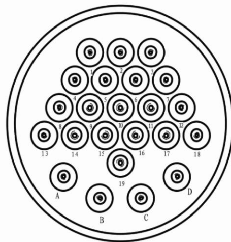
图6-2 隔爆型端子图
