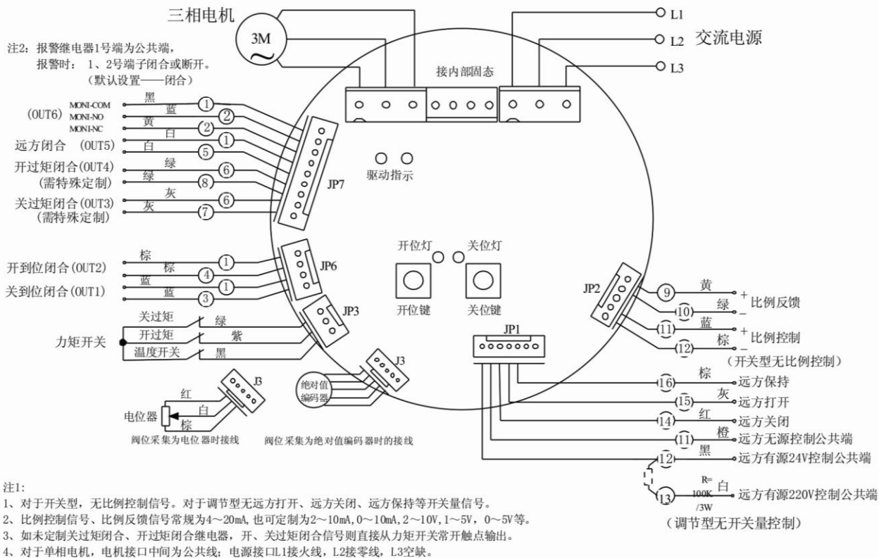
图5 内部连接图
