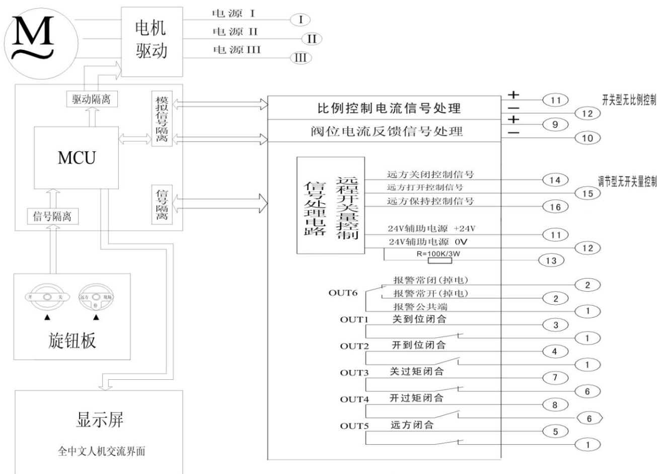
图4电气原理图
